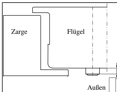
Überstandsmaß
