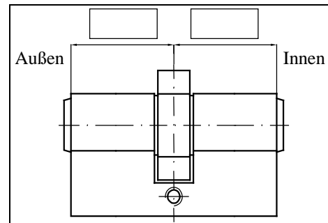
Abmessung Zylinder
