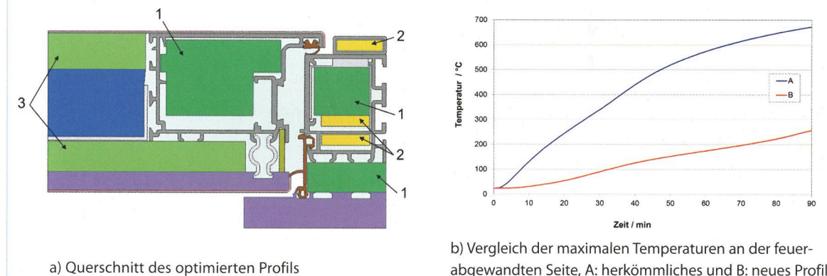
Bild 2: Simulation des Feuerwiderstands für Türrahmenvarianten.
